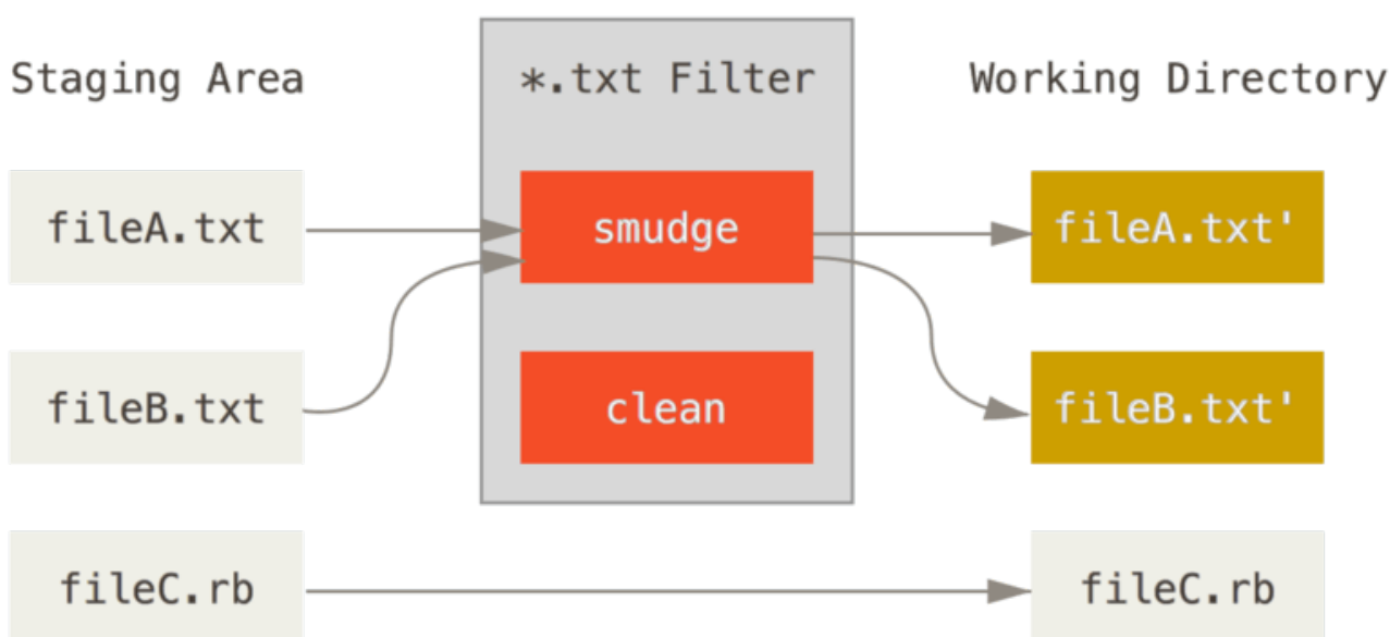
Figure 144. Ejecución de filtro “smudge” en el checkout.
