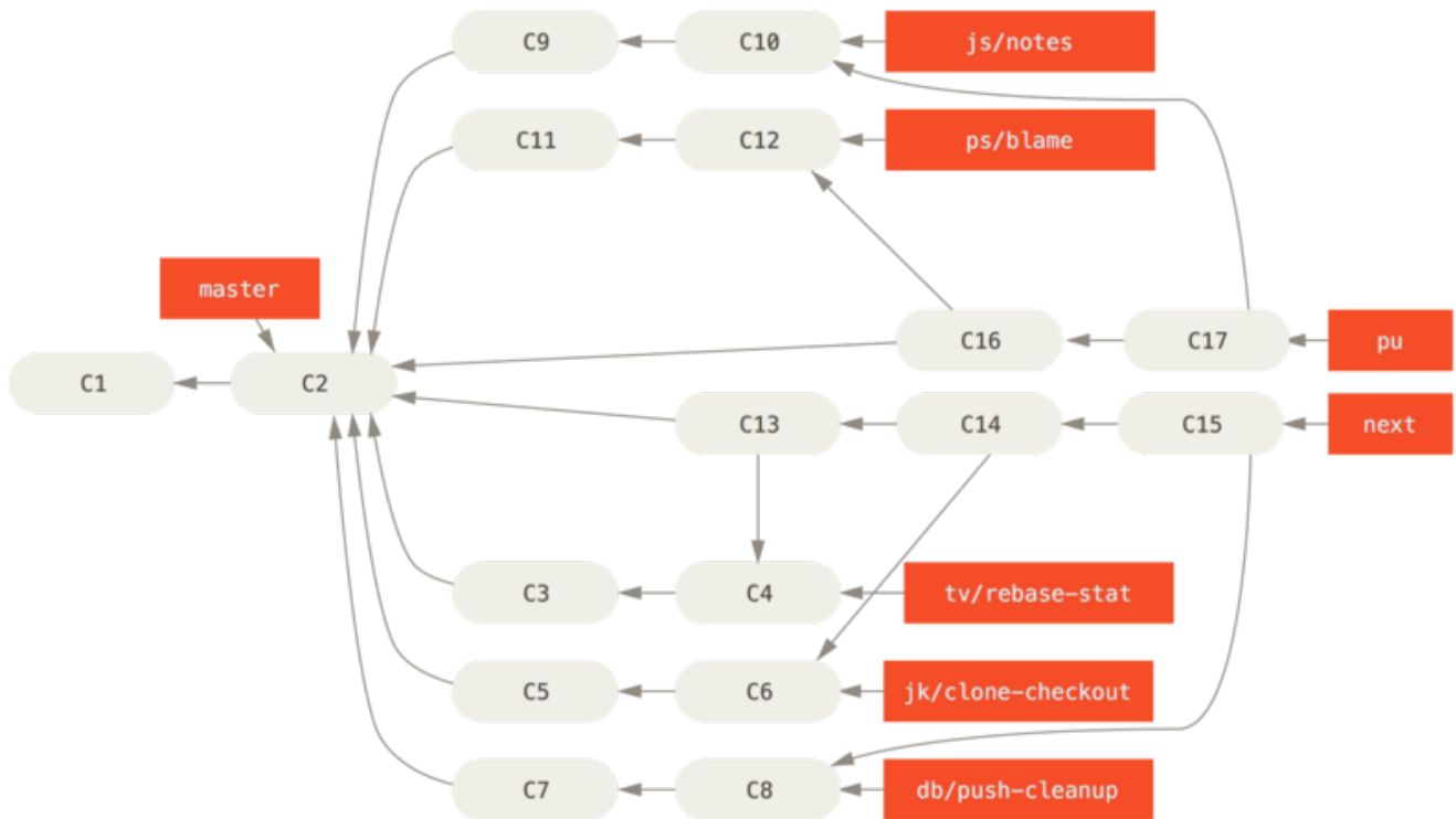
Figure 79. Fusionando ramas puntuales en ramas de integración de largo recorrido.
